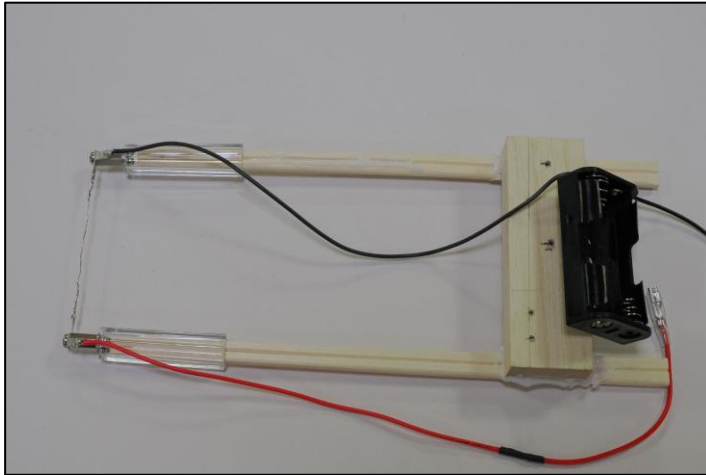
発泡スチロールカッター 完成イメージ
